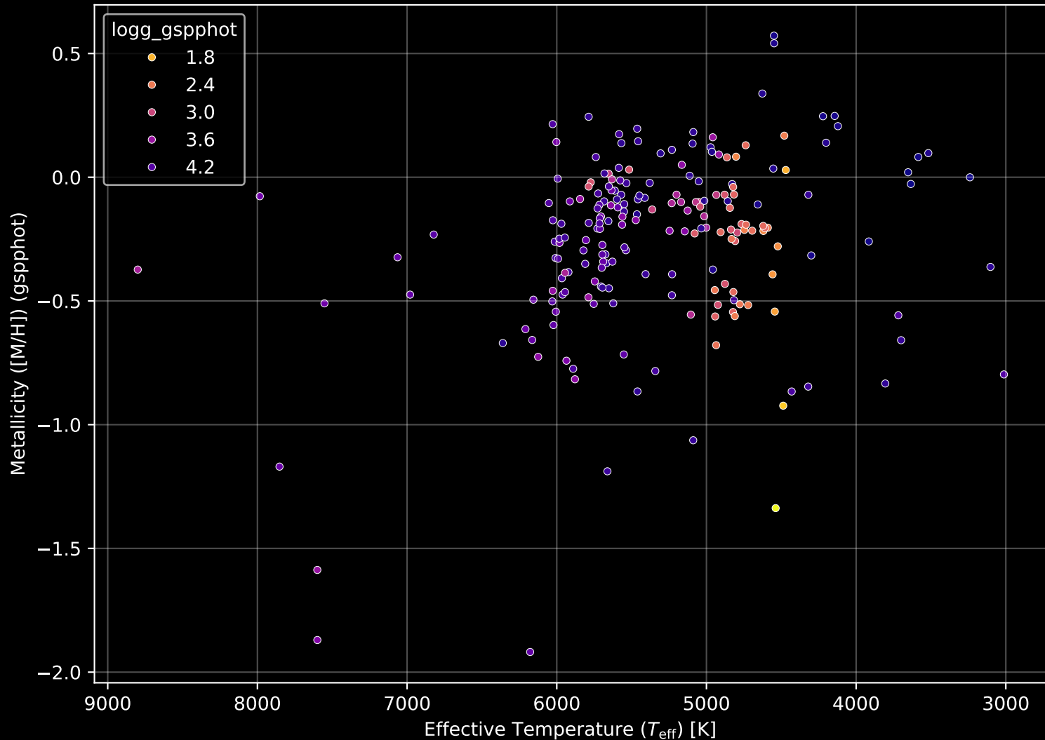
APOGEE DR17 Field: [230+32_MGA] Stellar Population Parameters (n= 204)
